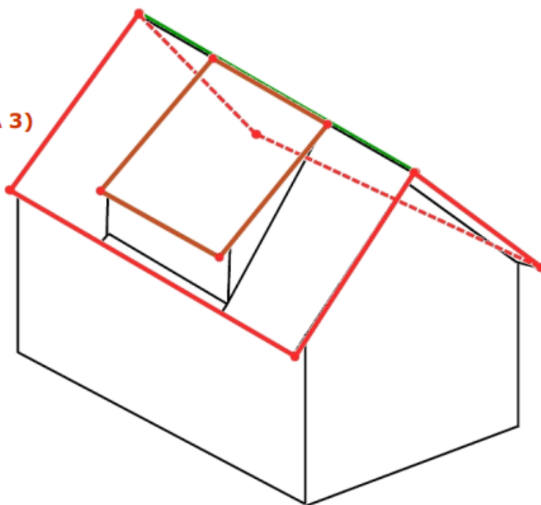
Figur 22. Eksempel på registrering av takoppbrett. Mønelinje og Bygningslinje skal registreres parallelt på topp møne. Her har mønelinja og bygningslinja ulikt TRE_D_NIVÅ og det skal derfor ikke lages nodepunkt i mønelinja. I tilfeller med takoppbrett på begge sider av mønet, skal disse ha en felles bygningslinje langs mønelinja.
