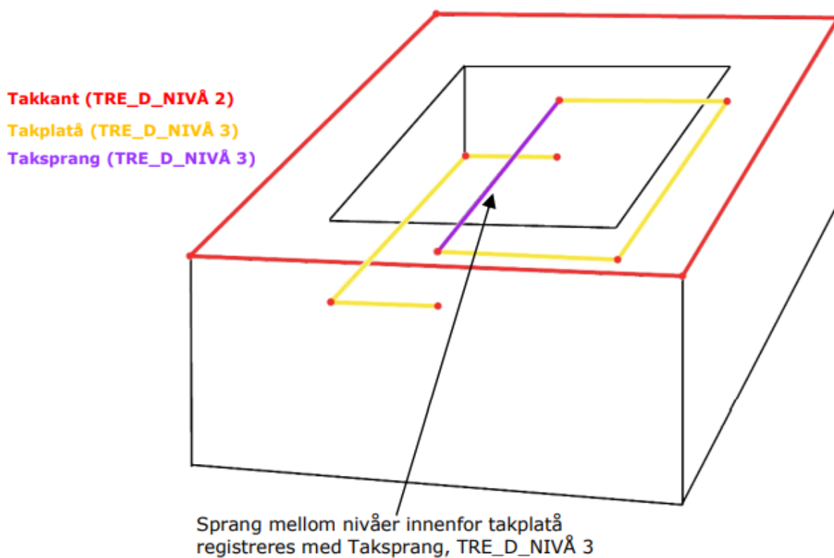
Figur 33. Eksempel på registrering av Takplatå i en bygård med indre rom
