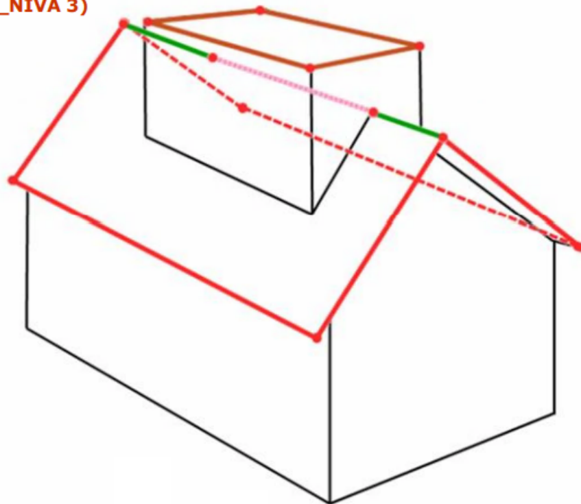
Figur 26. Eksempel på et bygg der man må benytte Hjelpelinje3D for å kunne beskrive hovedbygget fullstendig
