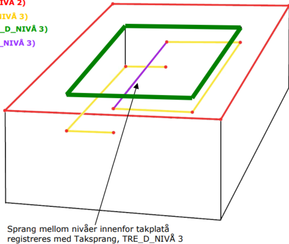
Figur 35. Eksempel på registrering av TakplatåTopp (mørk grønn linje)
