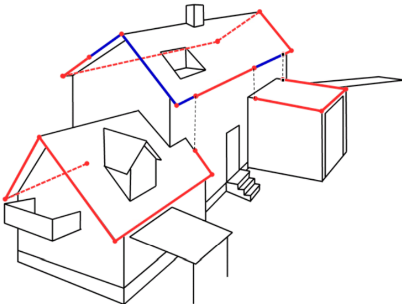
Figur 37. Eksempel på registrering av Taksprang (blå linje) og Takkant (rød linje).
