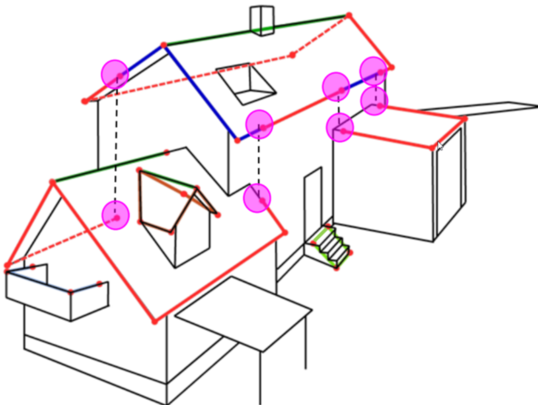
Figur 64. Eksempel på 2D-nodepunkt for en bygning. Disse er markert med en rosa ring.
