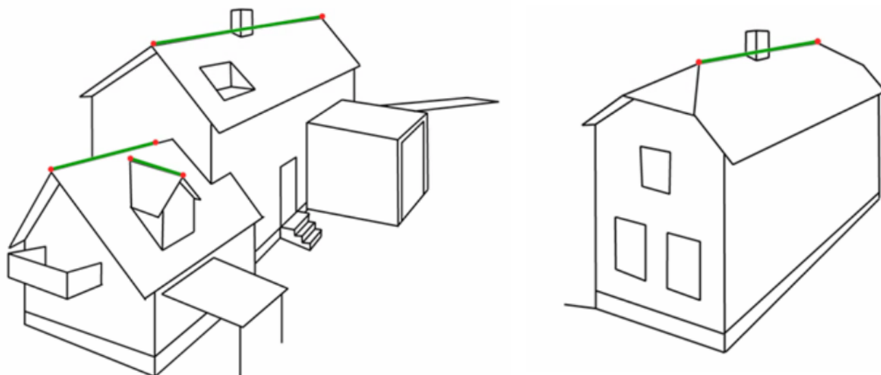
Figur 28. Eksempel på registrering av mønelinje. Mønelinje er tegnet grønt
