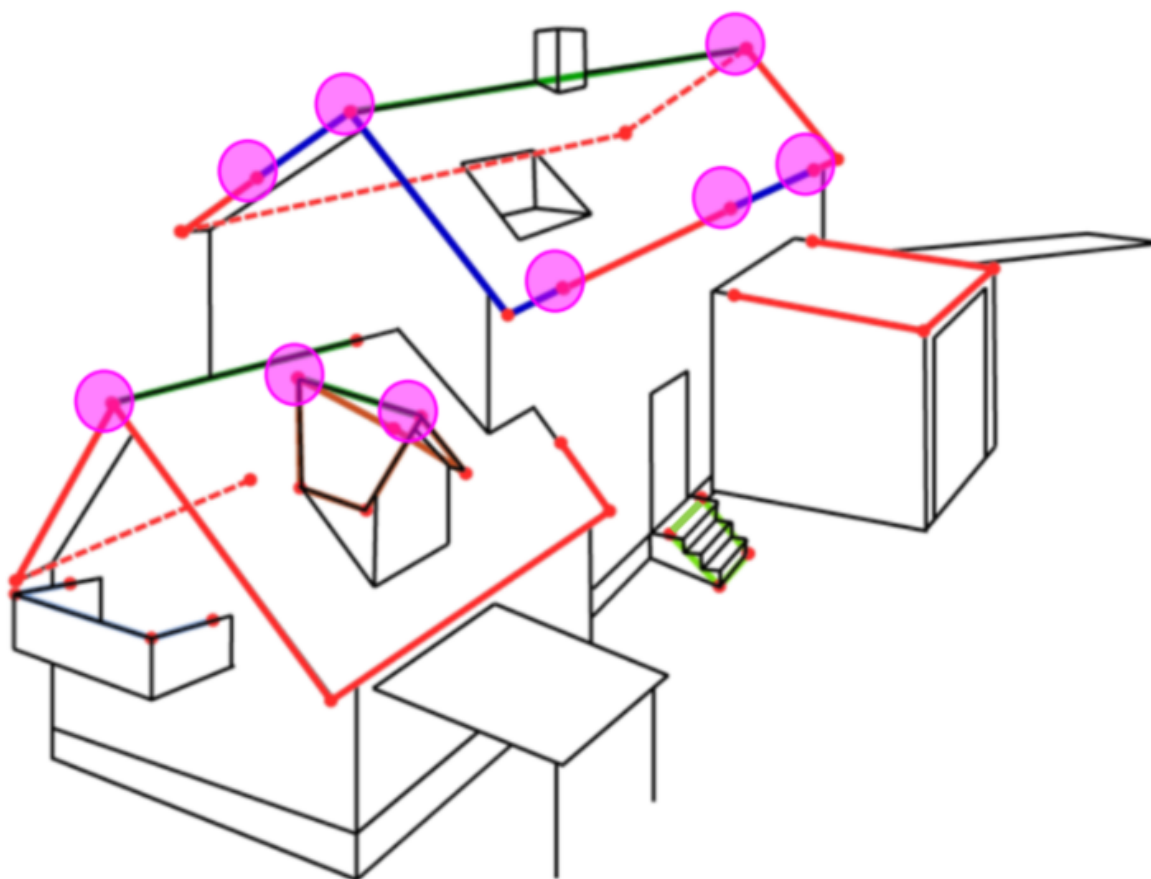
Figur 63. Eksempel på 3D-nodepunkt for en bygning. Disse er markert med en rosa ring. Røde linjer er takkant, mørkeblå linjer er taksprang, brune linjer er bygninglinjer og mørkegrønn linje er mønelinje.
