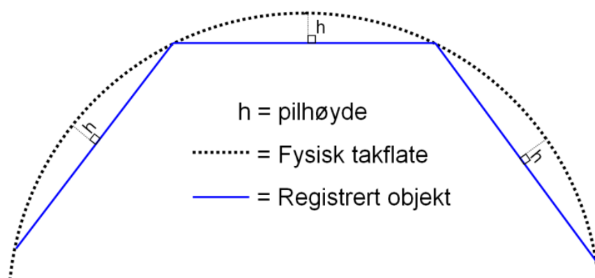
Figur 25. Prinsippskisser som viser bruk av Hjelpelinje3D for kuppel og spir. I figuren under vises hva som menes med pilhøyde. I de fleste tilfeller vil det være bunnen av den krumme flaten man må ta utgangspunkt i for å vurdere hvor tett det skal være med hjelpelinjer.
